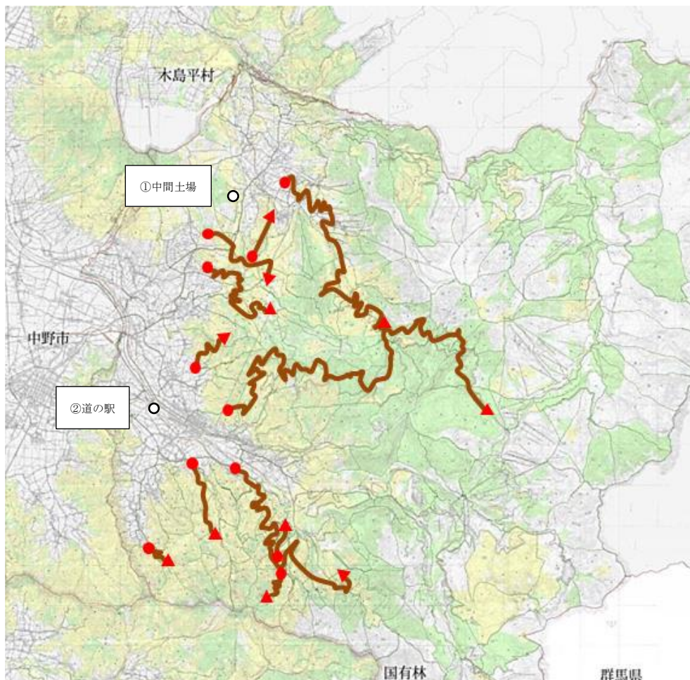
基幹路網位置図
